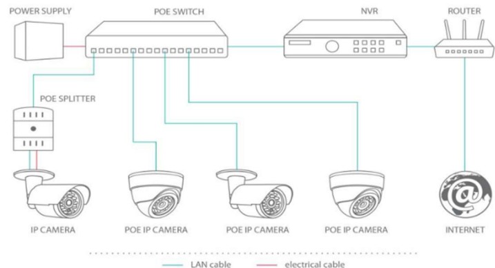
Схема підключення:
