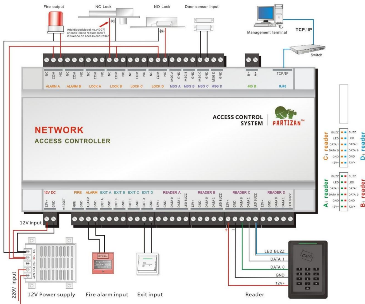
Fig.2. Esquema de conexión
