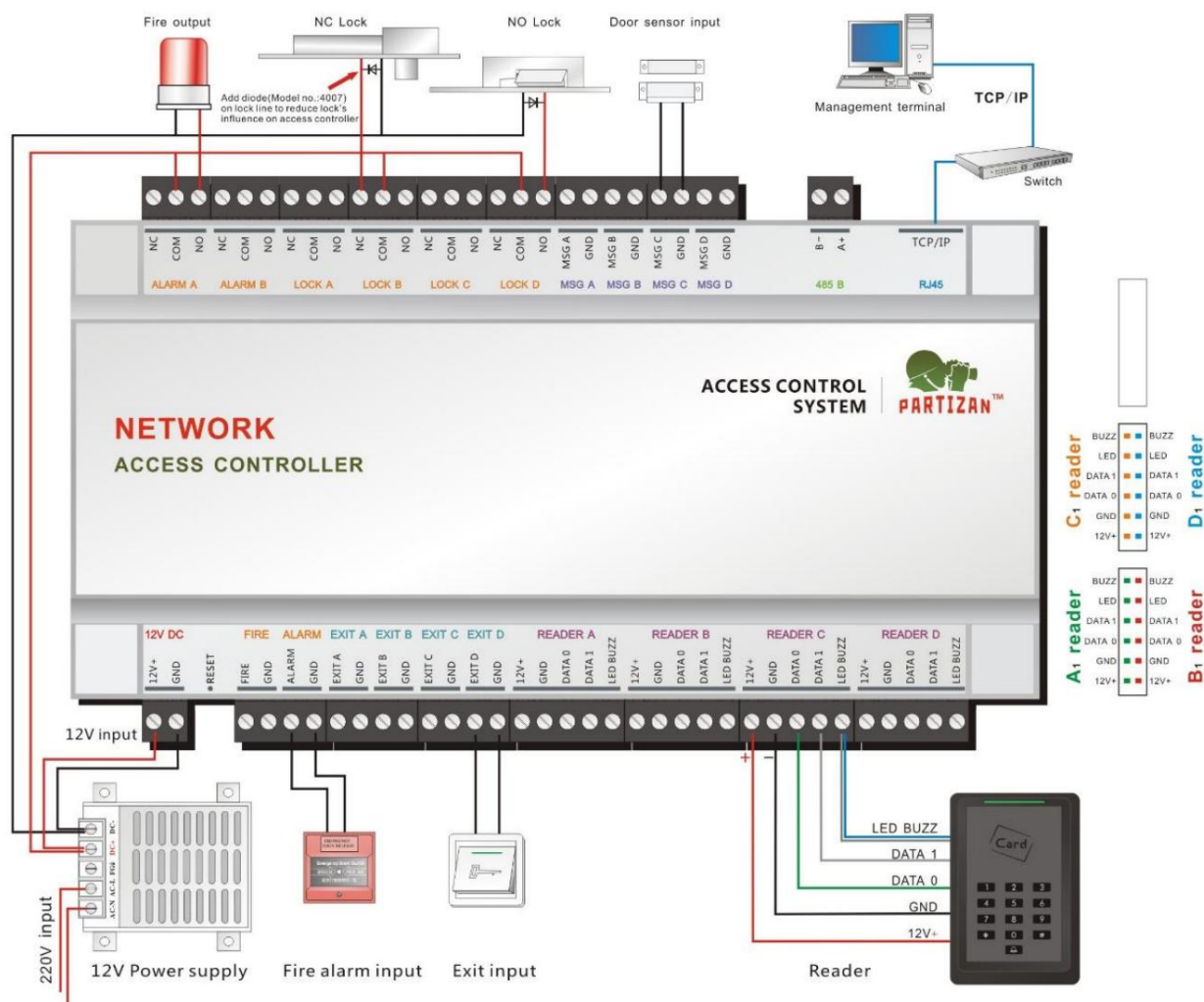
Fig.2. Schema di collegamento
