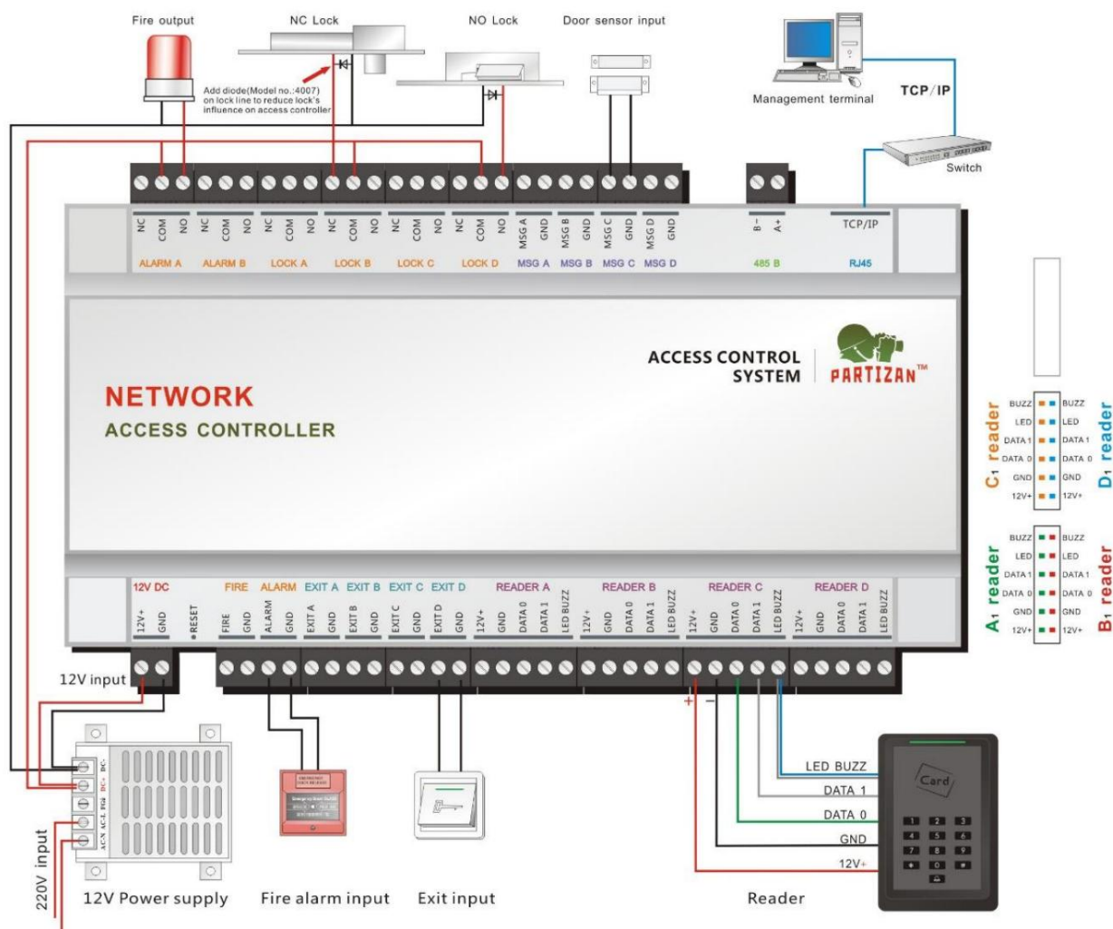
Мал.2. Схема підключення
